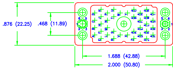
38 PIN RECEPTACLE
