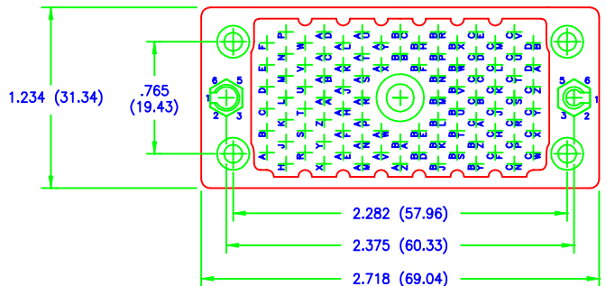
120 PIN RECEPTACLE
