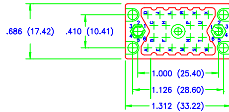
20 PIN RECEPTACLE
