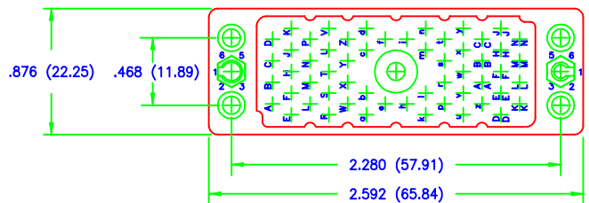
56 PIN RECEPTACLE
