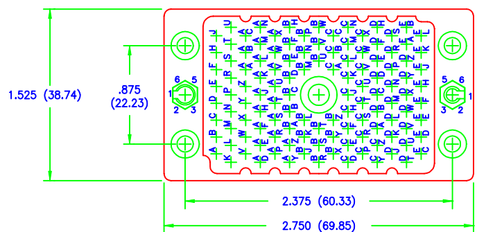
120 PIN RECEPTACLE
